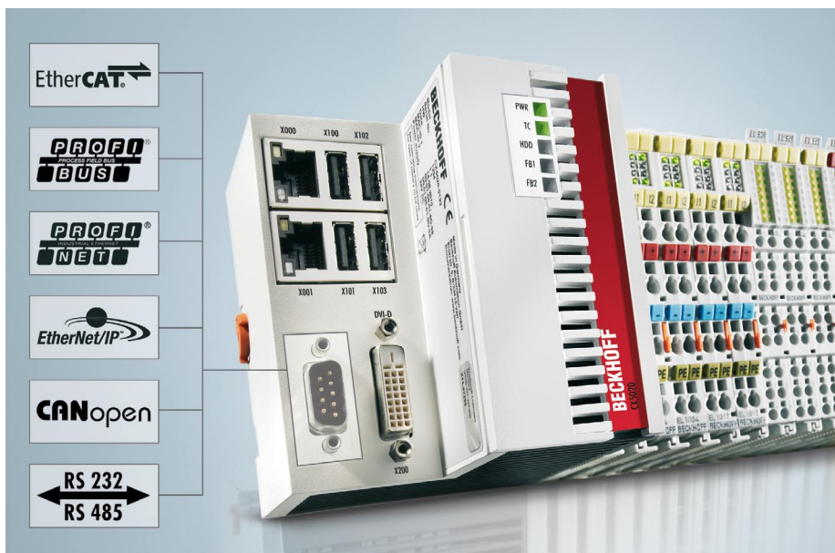
CX5020 Embedded PC met krachtige en energiezuinige Intel Atom 1,6 GHz processor
